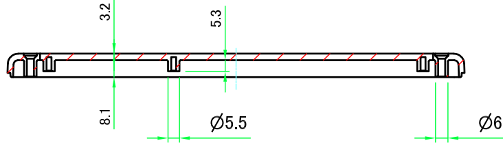
D-D ( 1 : 2.5 )
